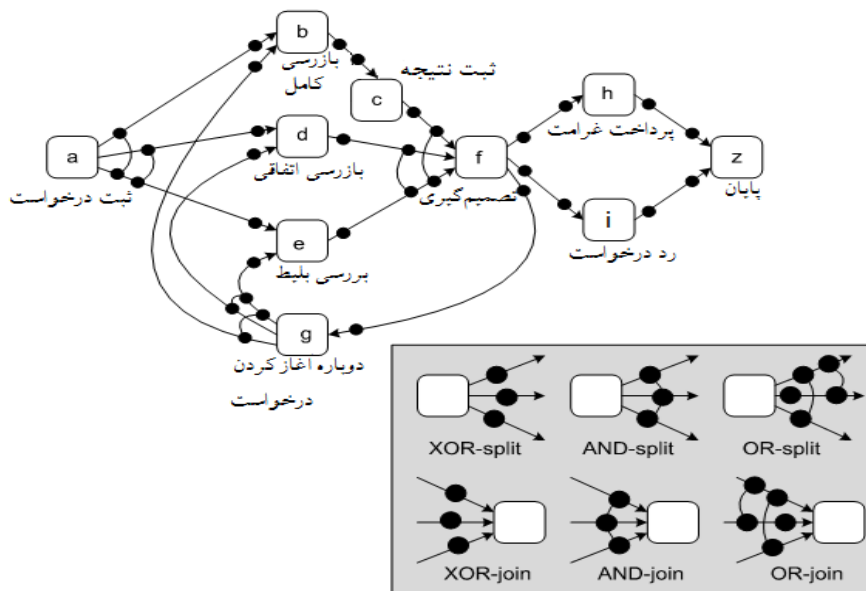
شکل ۱: شبکه علی فرآیند رسیدگی به درخواست‌های پرداخت گرامت در یک شرکت بیمه
