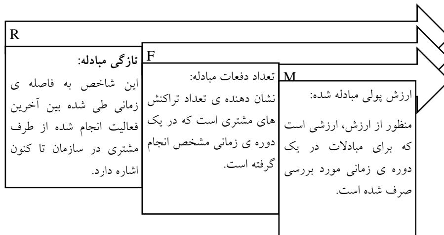
شکل ۱. مدل RFM
