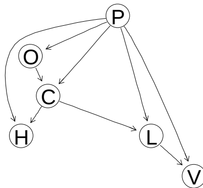
شکل ۳. ساختار تولید شده برای داده‌های هفتگی پس از آموزش ساختاری
