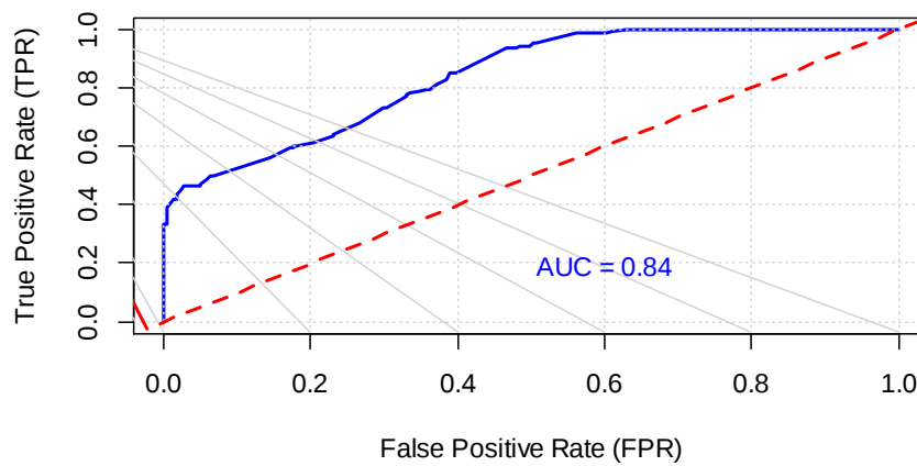
شکل ۷. نمودار منحنی ROC و مساحت زیر منحنی برای روش پیشنهادی در دستنمایی
